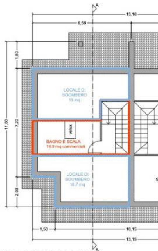
PIANTA PIANO SECONDO
