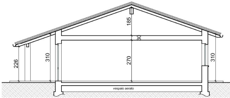
SEZIONE BB - sc. 1:100
