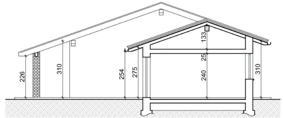
SEZIONE AA - sc. 1:100
