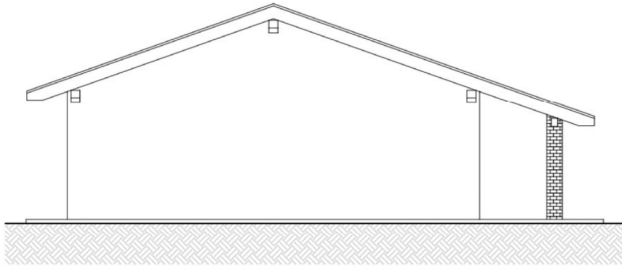
SEZIONE EST - sc. 1:100
